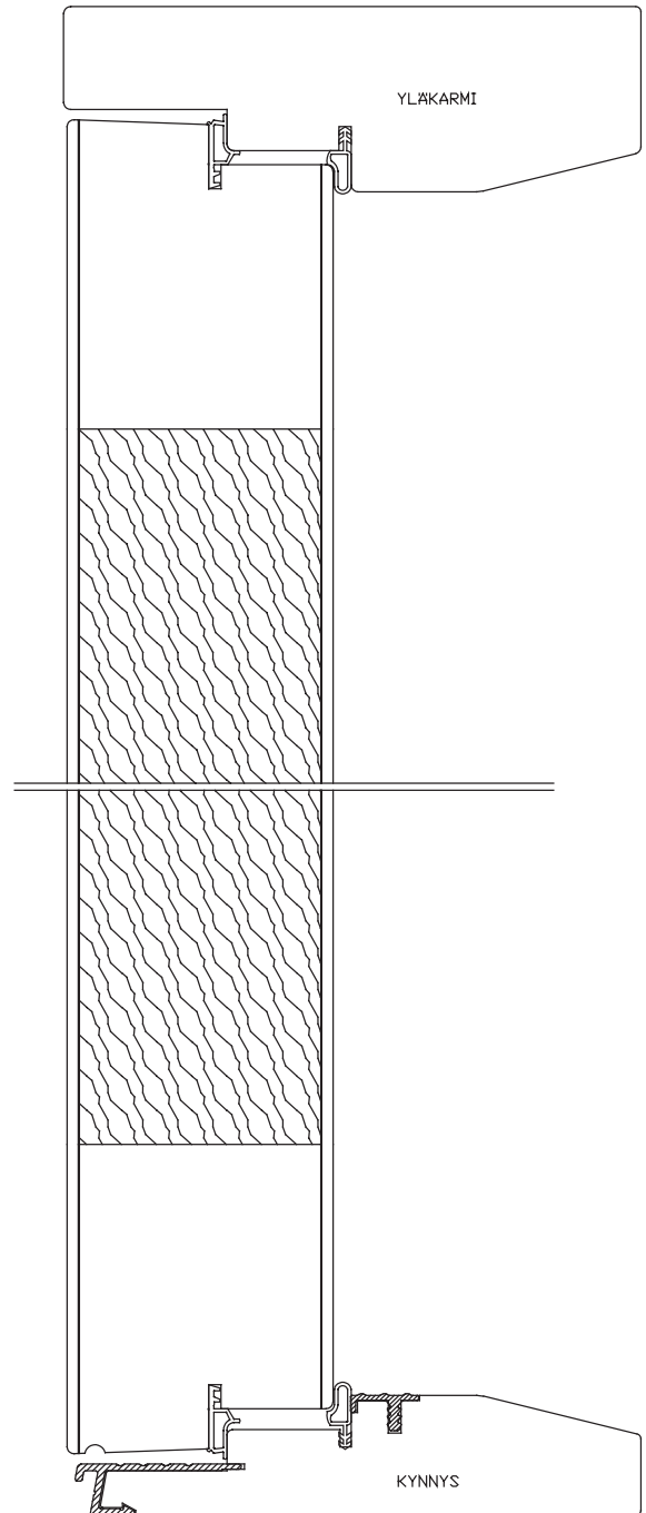
Pystyleikkaus, umpiovi
